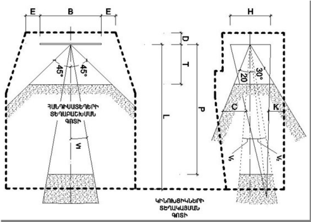
Գծապատկեր 1. Հանդիսասրահի, կինոթատրոնների և ունիվերսալ դահլիճների ցուցադրակրանի հարաչափերը
