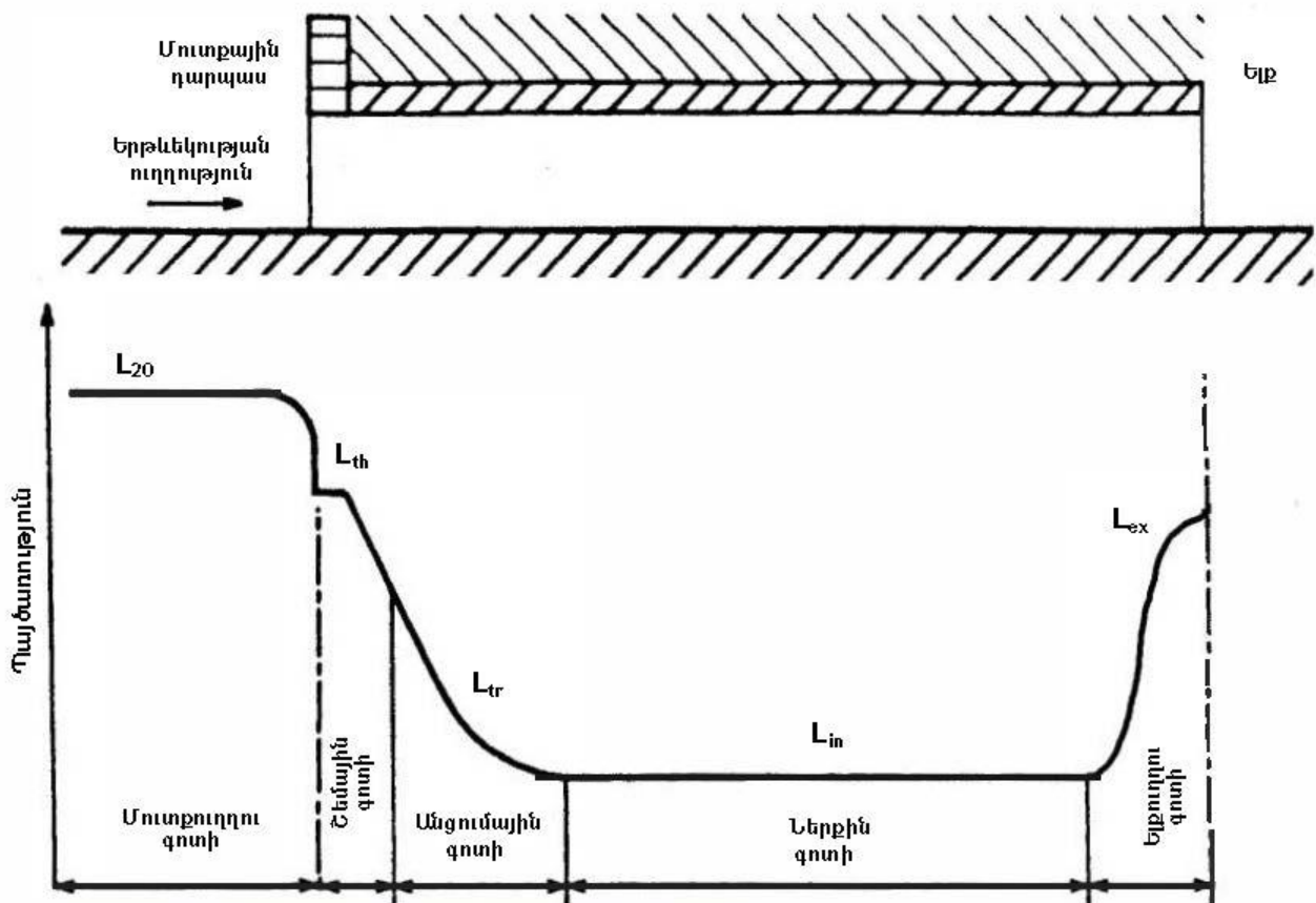
Գծապատկեր 1. Թունելի պայծառ գոտիները ցերեկային ռեժիմում
