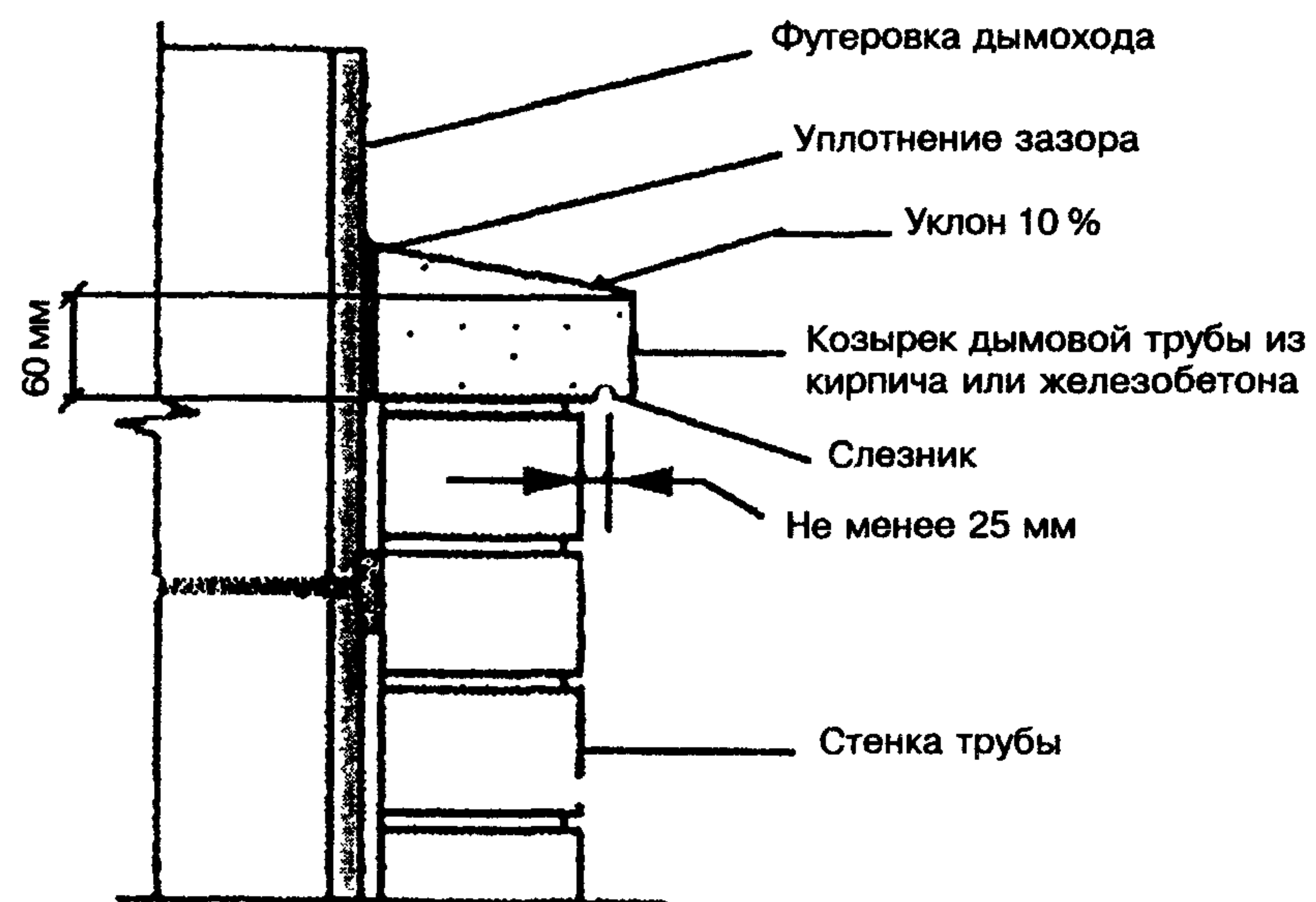
Рисунок 7.7 — Оголовок дымовой трубы
