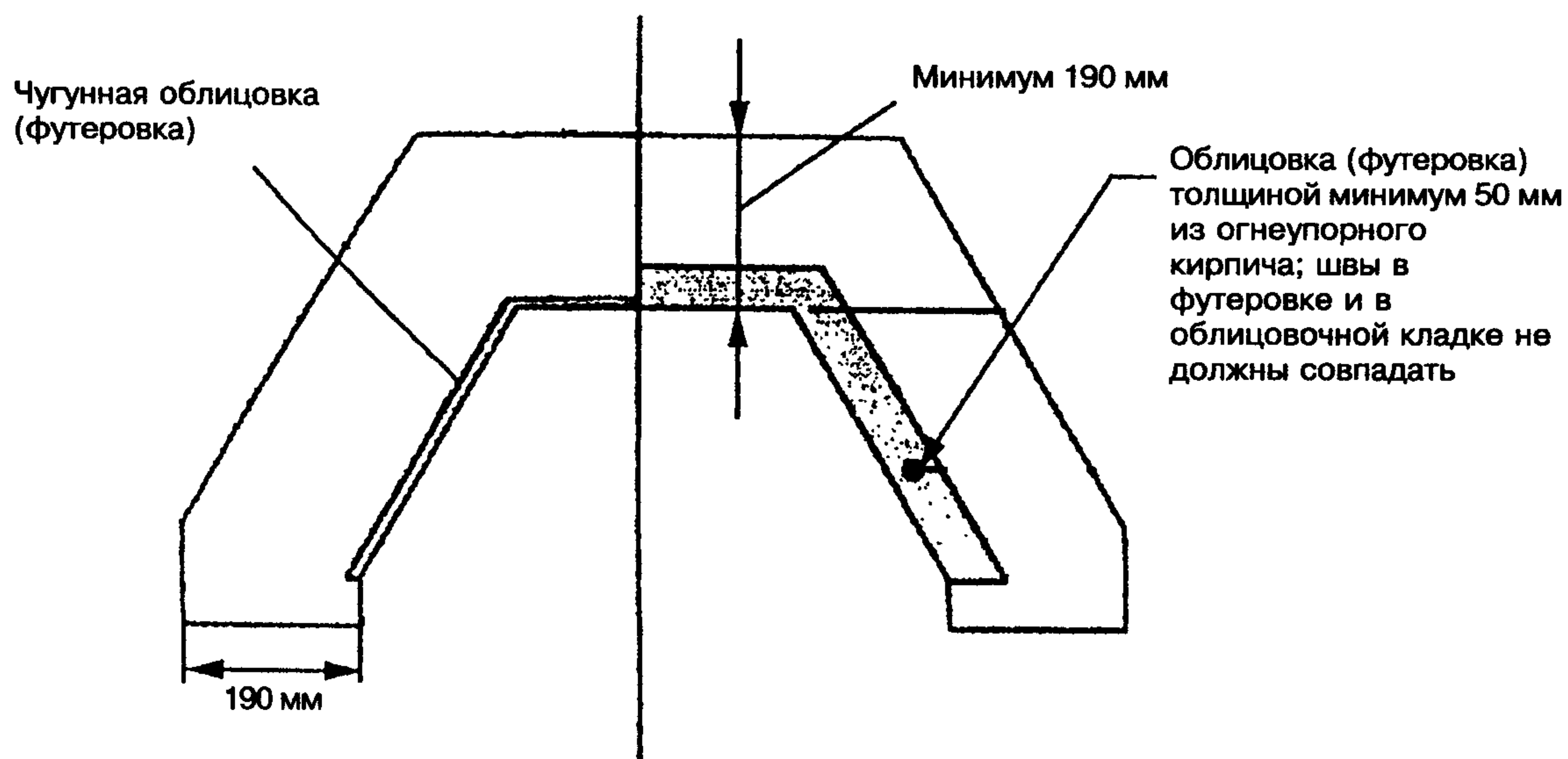
Рисунок 7.5 — Футеровка камина
