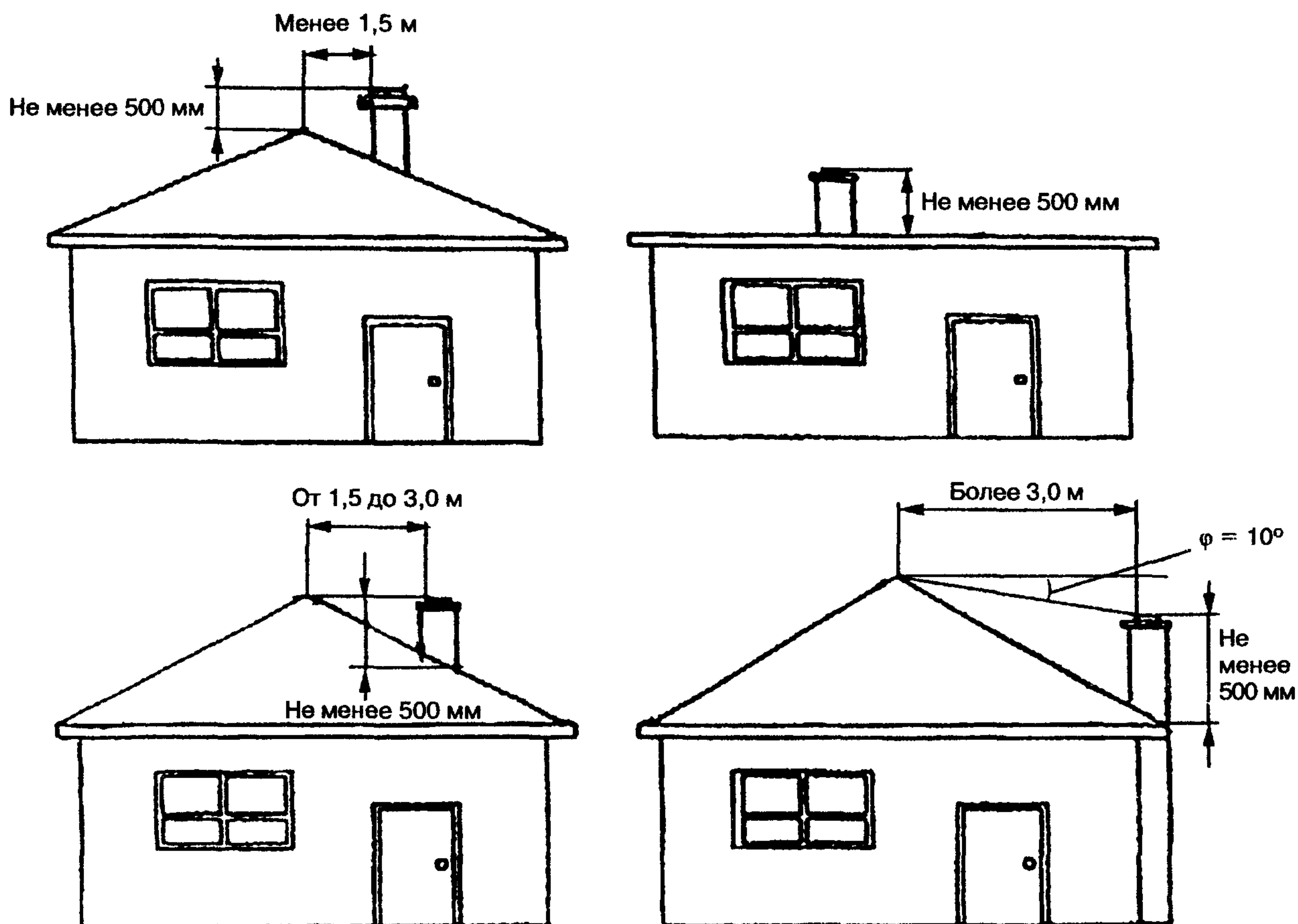
Рисунок 7.9 — Минимальная высота дымовой трубы
