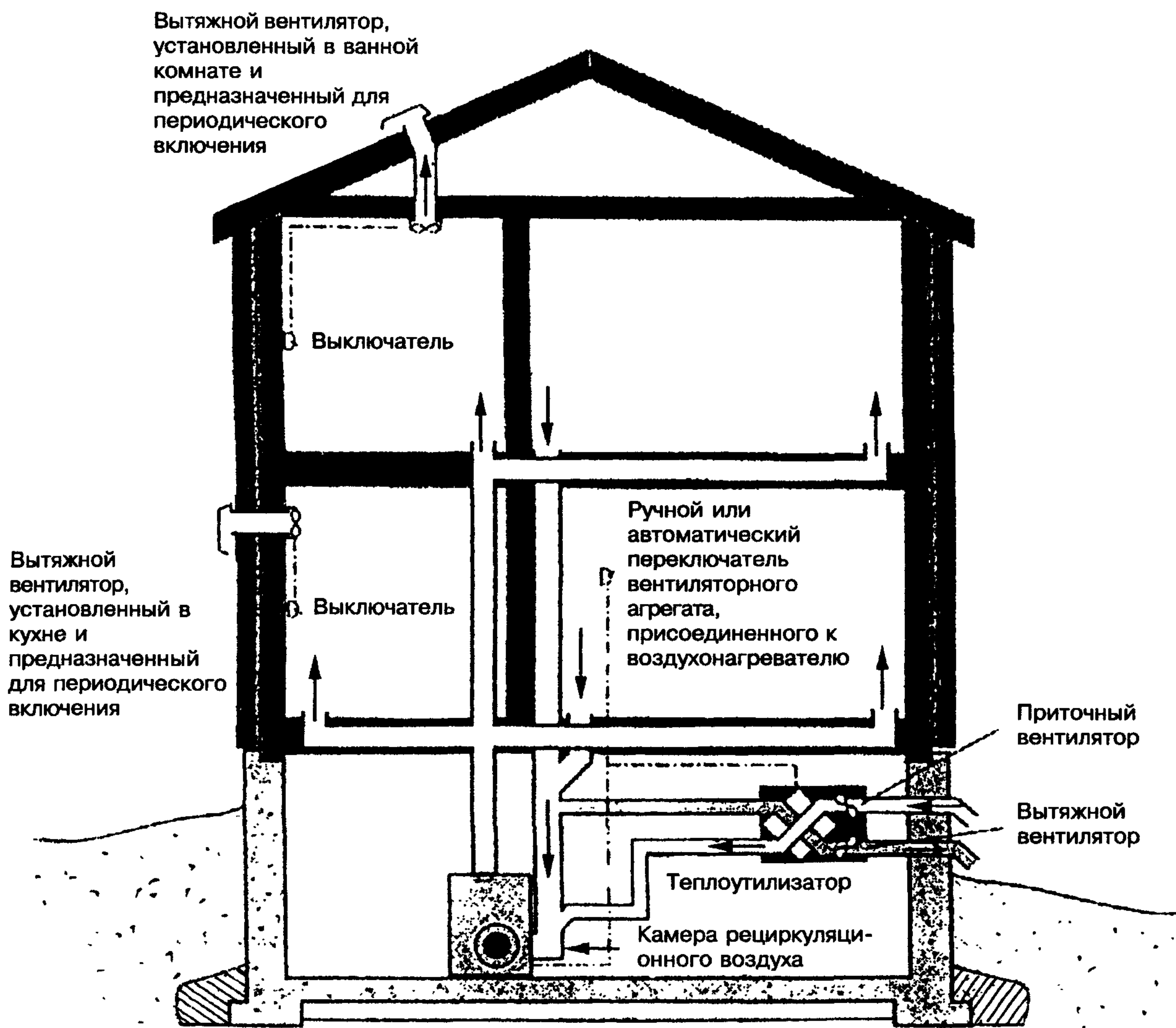
Рисунок 7.3 — Присоединение теплоутилизационного агрегата к камере подогрева воздуха
