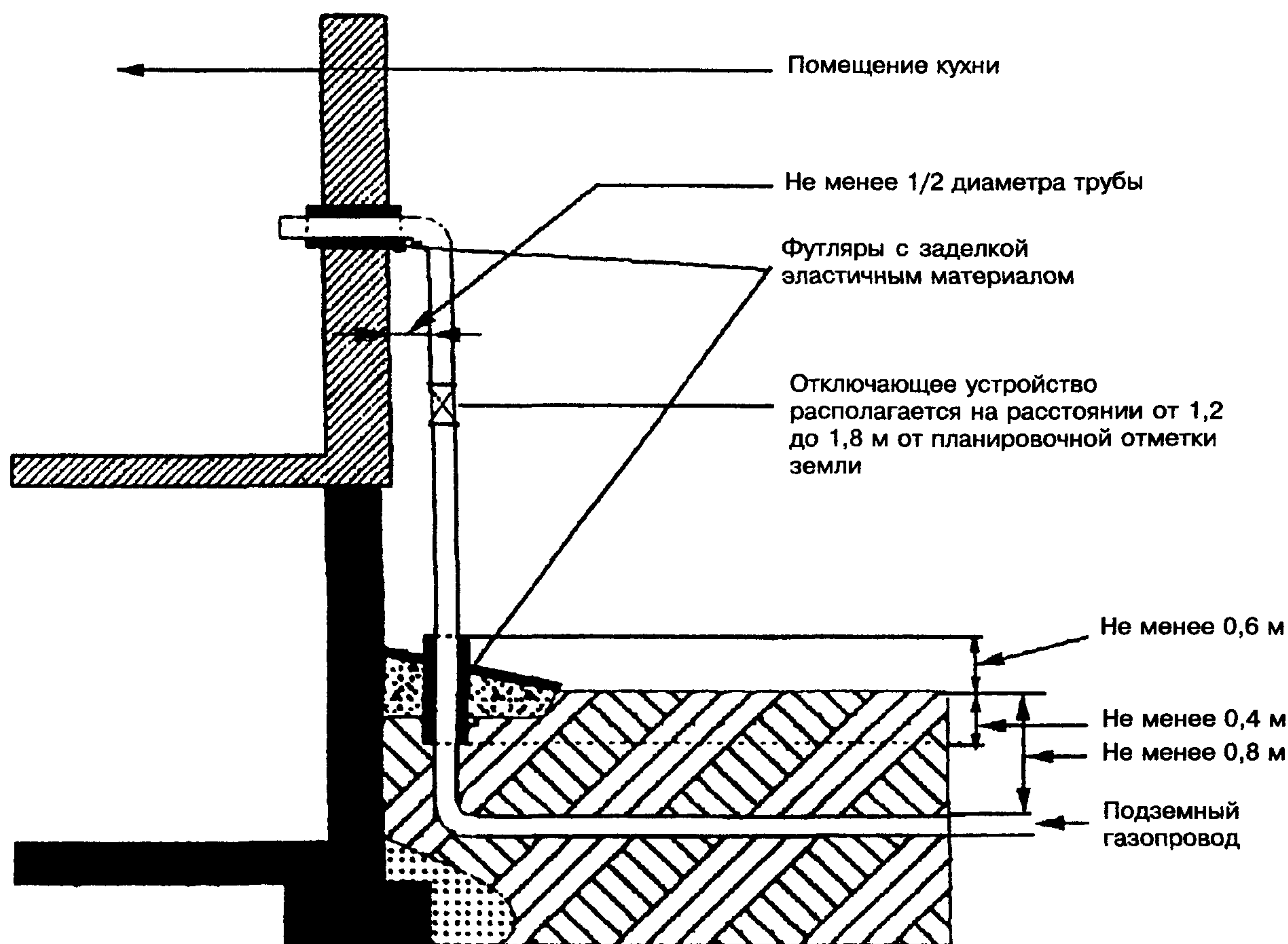
Рисунок 9.1 — Газовый ввод
