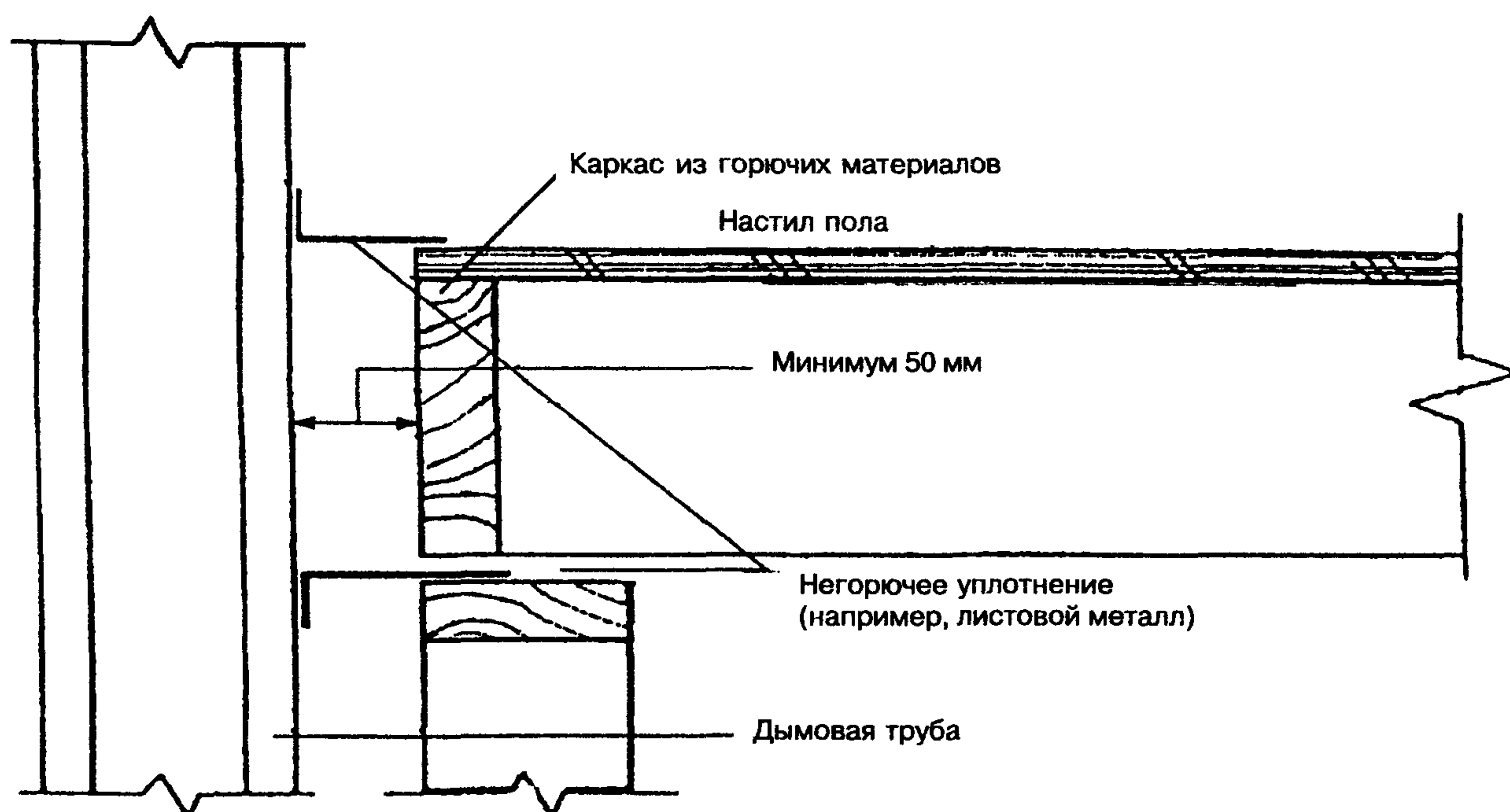
Рисунок 7.8 — Расстояние от дымовой трубы до строительных конструкций
