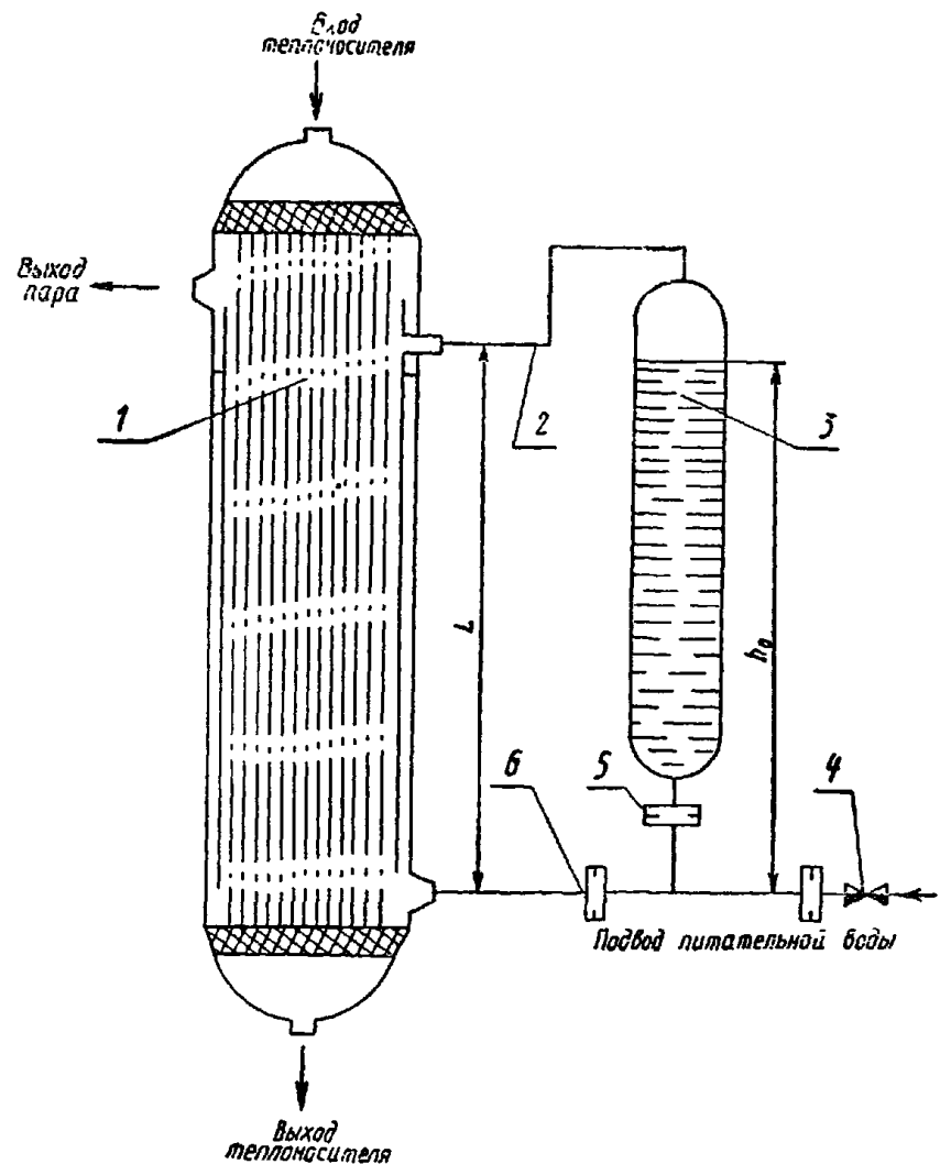
1 — парогенератор; 2 — паровой «дыхательный» патрубок; 3 — гидроемкость; 4 — регулирующий клапан; 5 — дроссель гидроемкости; 6 — дроссель на входе в парогенератор
