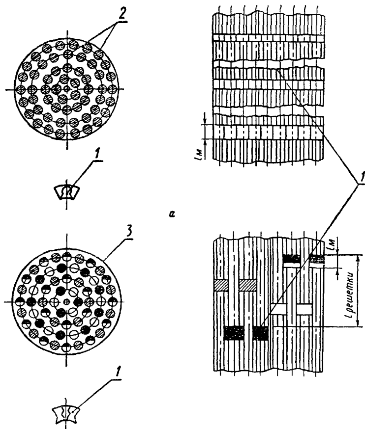
1 — дистанционирующие муфты; 2 — трубки; 3 — канал
