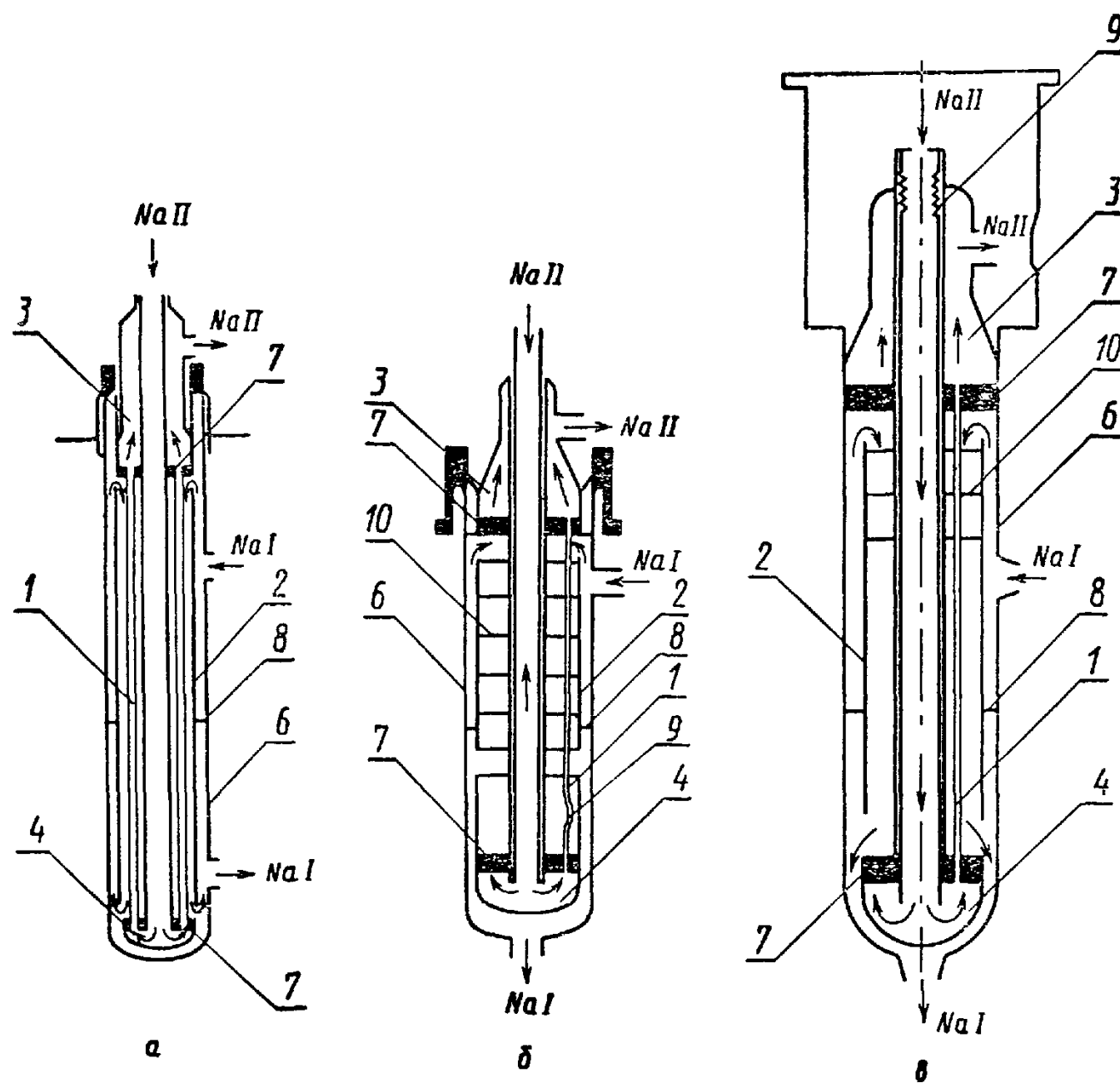
а — ПТО реактора SNR 300 б — ПТО реактора FFTF в — ПТО реактора CRFBR, 1 — трубный пучок, 2 — обечайка 3 — верхний коллектор 4 — нижний коллектор 5 — корпус 6 — трубная доска 7 — уплотнение 8 — компенсатор 9 — дистанционирующая решетка NaI — натрий первого контура NaII — натрий второго контура
