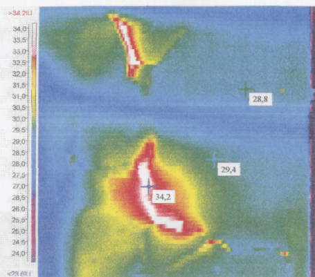
Рис.2.1 Разрушение футеровки котла (трещина) (калибровка шкалы в инструментальных единицах)
