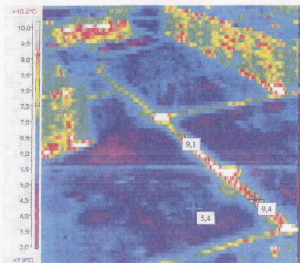
Рис. 5.10 Затопленный участок подземной теплотрассы (съемка с вертолета)
