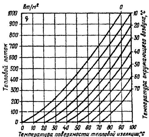
Номограмма для коэффициента излучения поверхности C=2,67 Вт/(м К)
