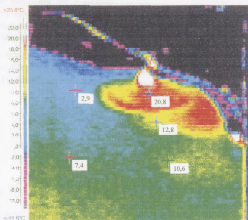
Рис. 6.2 Распределение температур на поверхности пруда охладителя ТЭЦ
