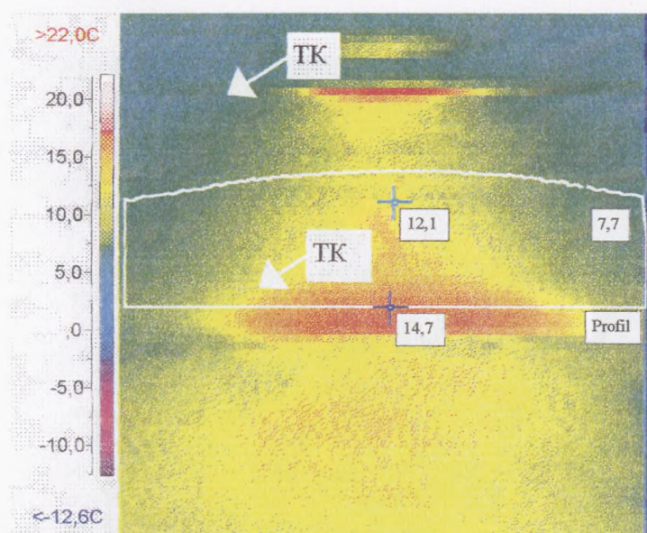
Рис. 5.9 Участок теплотрассы без дефектов
