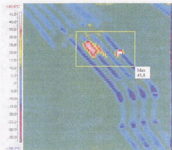
Рис. 5.11 Участок теплотрассы надземной прокладки с нарушением изоляции (Съемка с вертолета)
