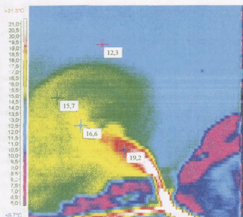
Рис. 6.1 Распределение температур на поверхности пруда охладителя ТЭЦ
