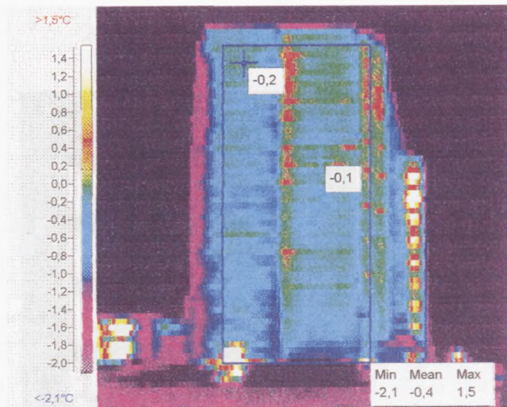
Рис. 1-9 Торцевая часть 9-ти этажного здания. Поверхность с t = -0,4\text{ }^{\circ}\text{C} , можно принять за базовый участок. Красная полоса в центре здания вызвана тепловым отражением.
