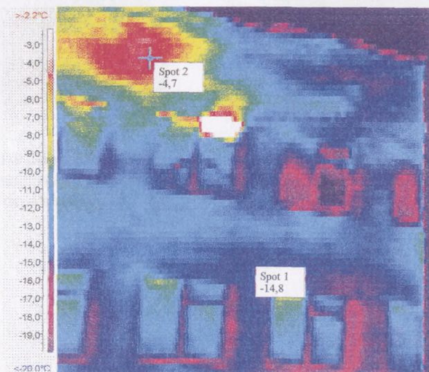
Рис.1.8 Термограмма малоэтажного кирпичного здания. В верхней части участок с повышенными теплопотерями. Фрагмент стены с температурой -14,8^{\circ}\text{C} здесь принят, как базовый.
