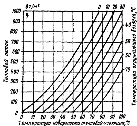
Номограмма для коэффициента излучения поверхности C=4,88 Вт/(м К)
