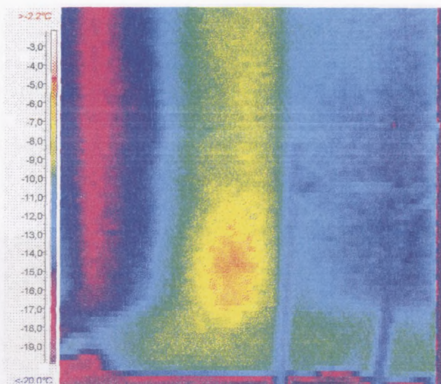
Рис.1.7 Участок стены сооружения с повышенными теплопотерями. (Его границей следует считать изотерму -11^{\circ}\text{C} )
