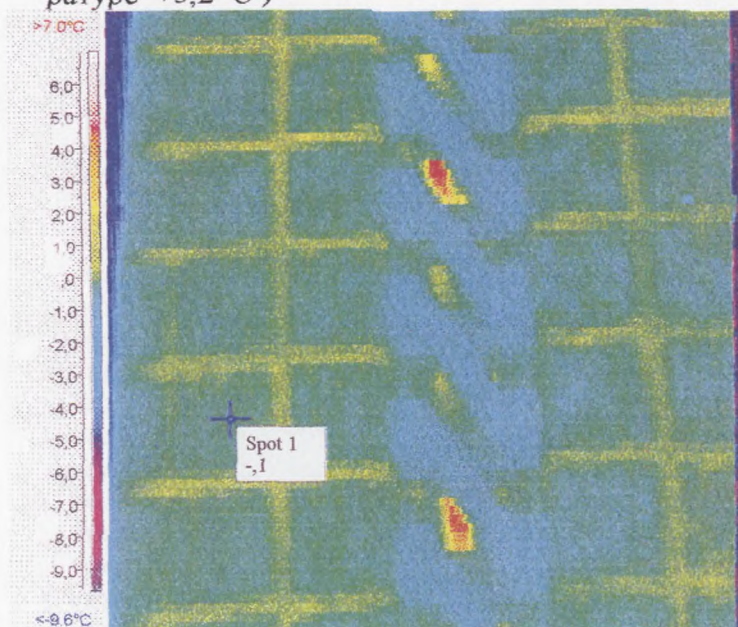
Рис.1.6 Термограмма стены панельного здания без оконных проёмов. Участок с температурой -3^{\circ}\text{C} может быть принят как базовый.
