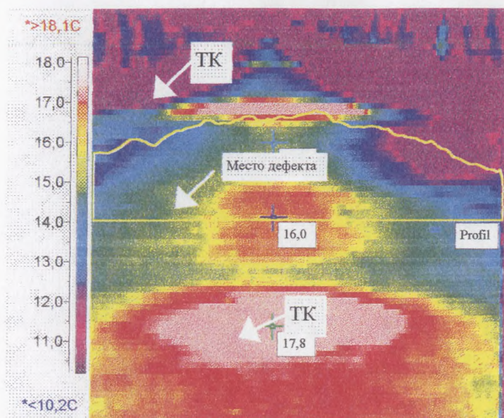
Рис. 5.8 Участок подземной теплотрассы с нарушенной изоляцией.
