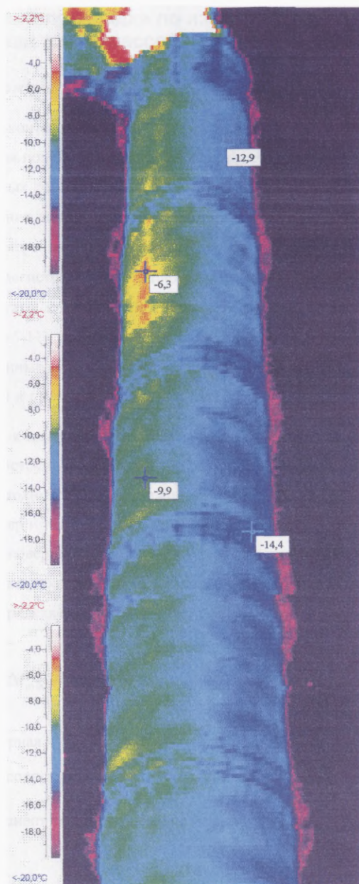
Фрагмент верхней части железобетонной дымовой трубы. Н=180 м
