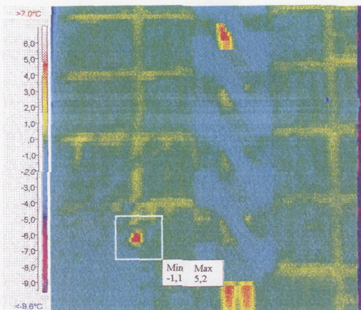
Рис.1.5 Термограмма стены панельного здания без оконных проёмов. В левой части видно место воздухопроница- ния через межпанельный шов. (Соответствует темпе- ратуре +5,2^{\circ}\text{C} )
