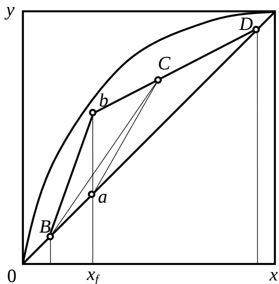
Рис. 2.19. Влияние изменения температуры питания
