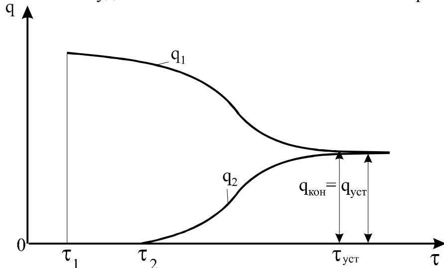
Рис. 1.15. Характер изменения удельных тепловых потоков
