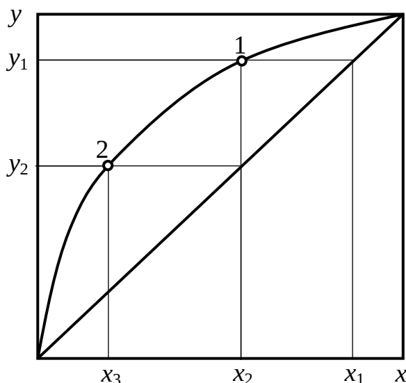
Рис. 2.17. К выводу уравнения Фенске
