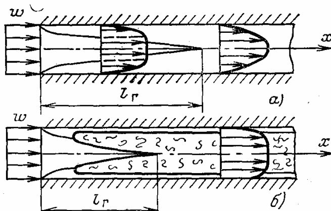
Рис. 1.8. Гидродинамическая стабилизация в трубе при ламинарном (а) и турбулентном (б) течениях
