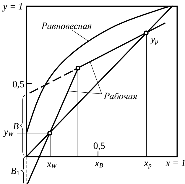
Рис. 2.16. Рабочая и равновесная линии в процессе ректификации
