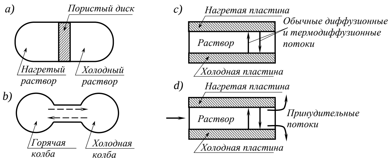
Рис. 2.32. Схемы термодиффузионных аппаратов, работающих по статическому методу
