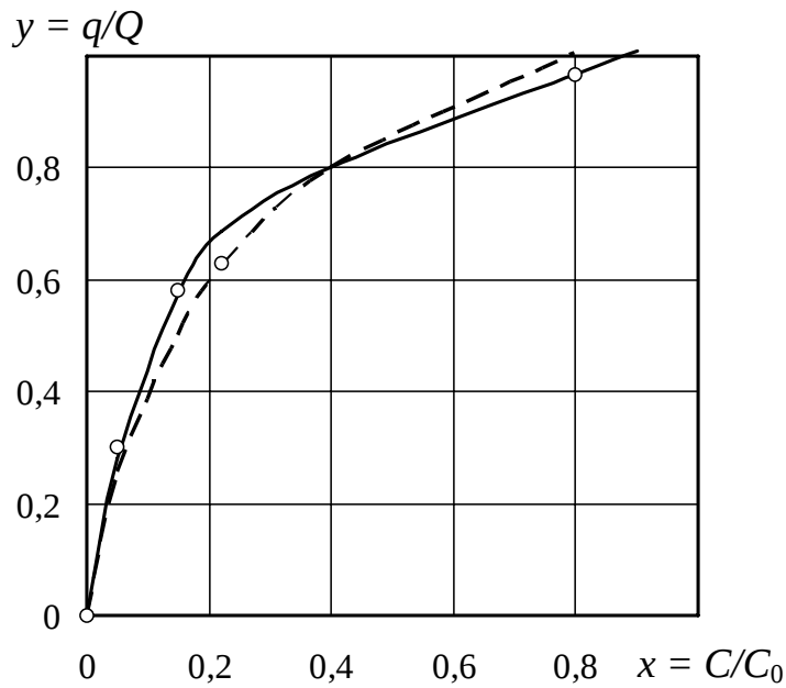
Рис. 2.23. Приближение к экспериментальному равновесию с помощью кривой фактора разделения r
